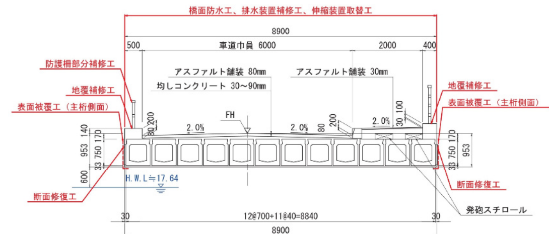
標準断面図
