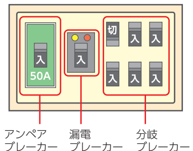
分電盤の例
