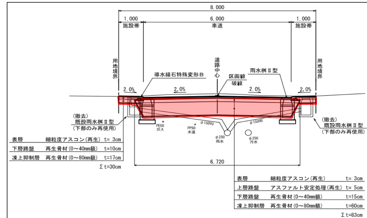
【断面図】
