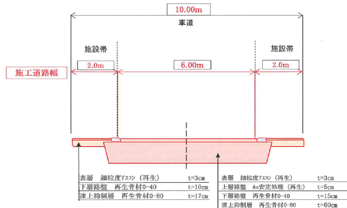
【断面図】
