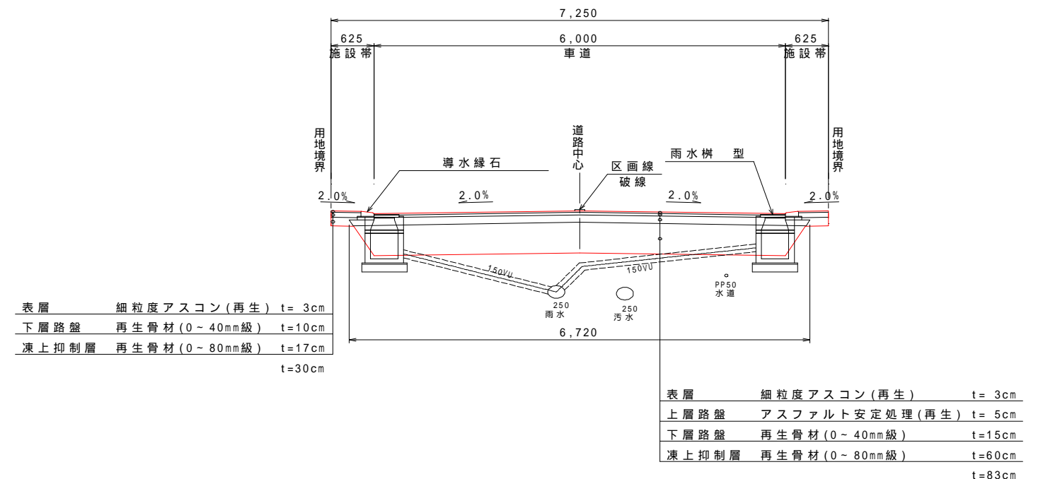
【 標 準 断 面 図 】
