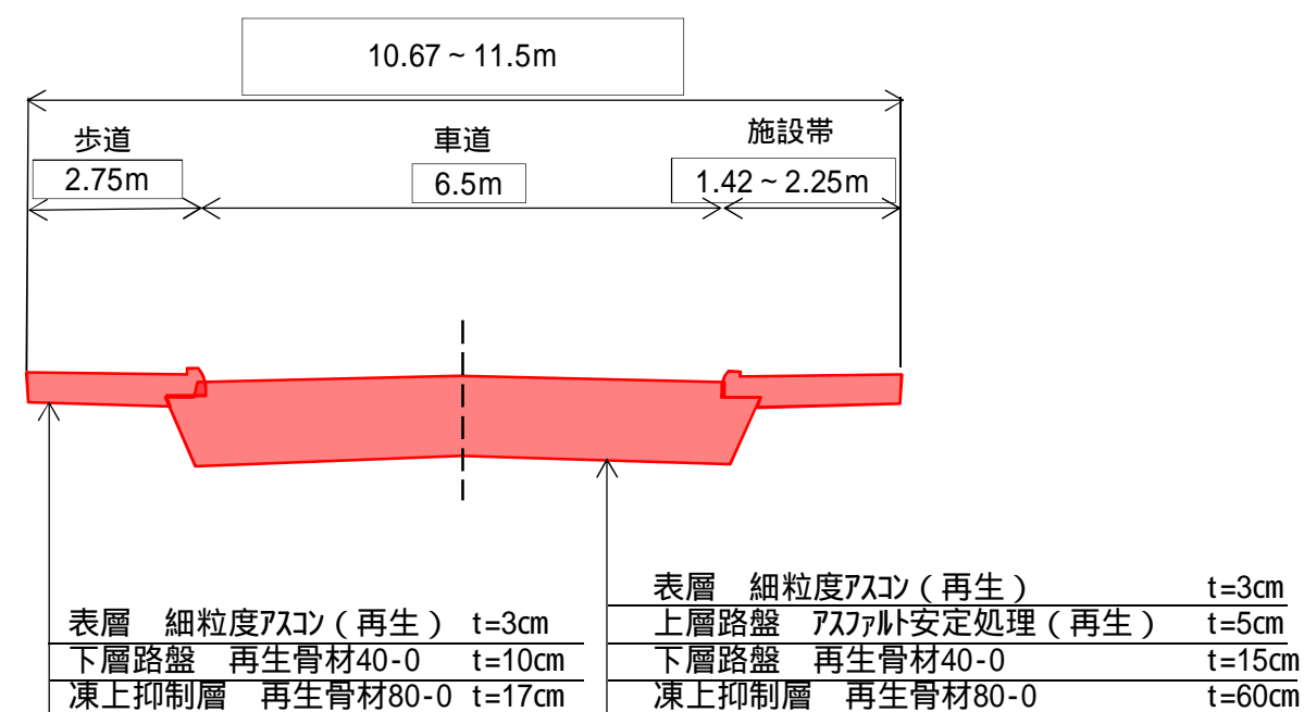
【断面図】
