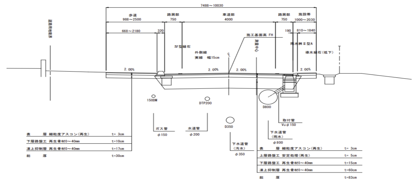
【標準断面図】
