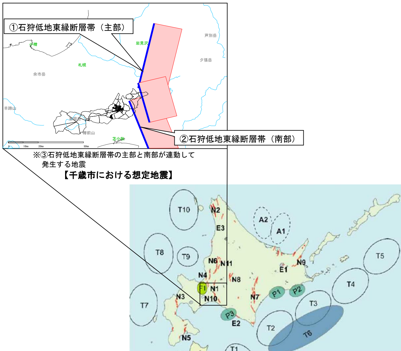
図3-1 北海道で想定される地震 ※出典：北海道地域防災計画
