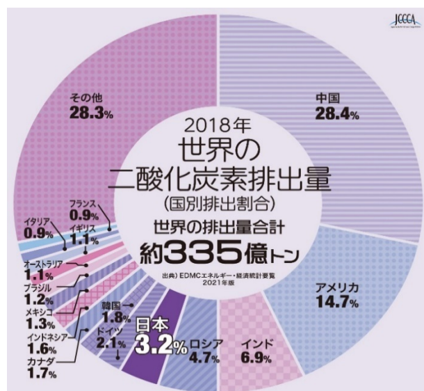
図 6 - 2 世界の二酸化炭素の国別排出量（2018 年）
