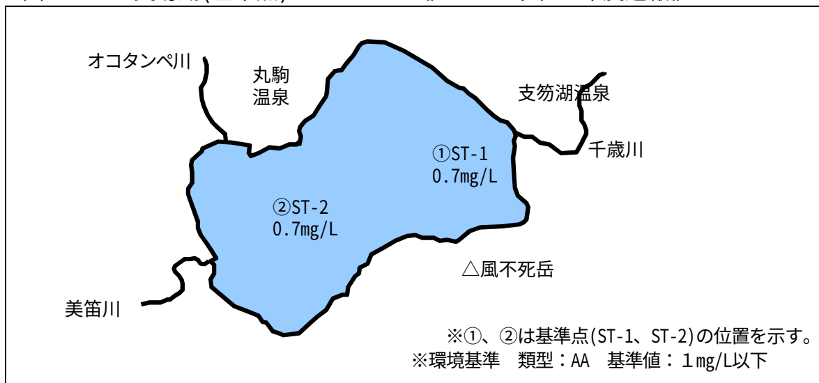
図3-12 支笏湖（基準点）のCODの75%値 令和2年度速報値
