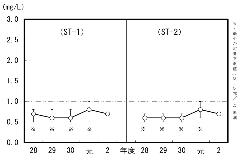
図3-11 CODの経年変化（支笏湖） 令和2年度は速報値
