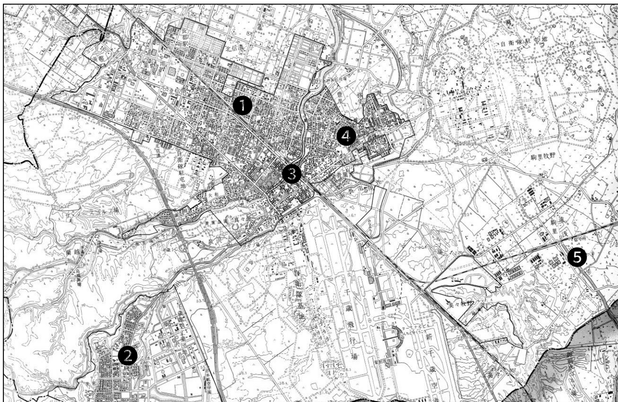
図3-2 大気汚染物質測定局位置図
