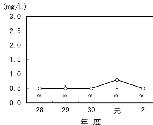
図3-5 BODの経年変化(祝梅川)
