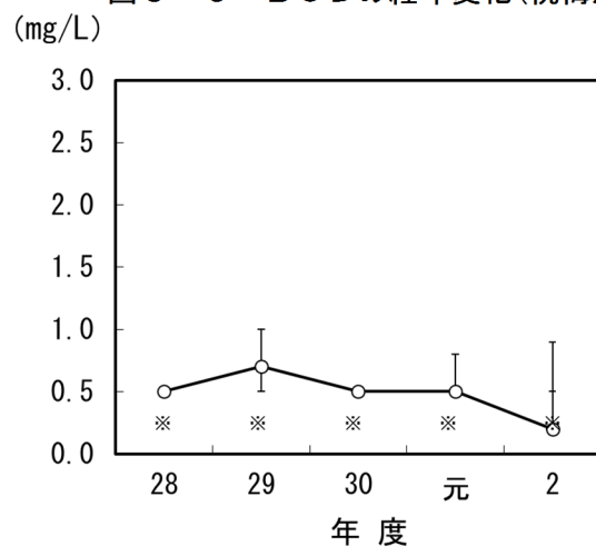
図3-5 BODの経年変化(祝梅川)
