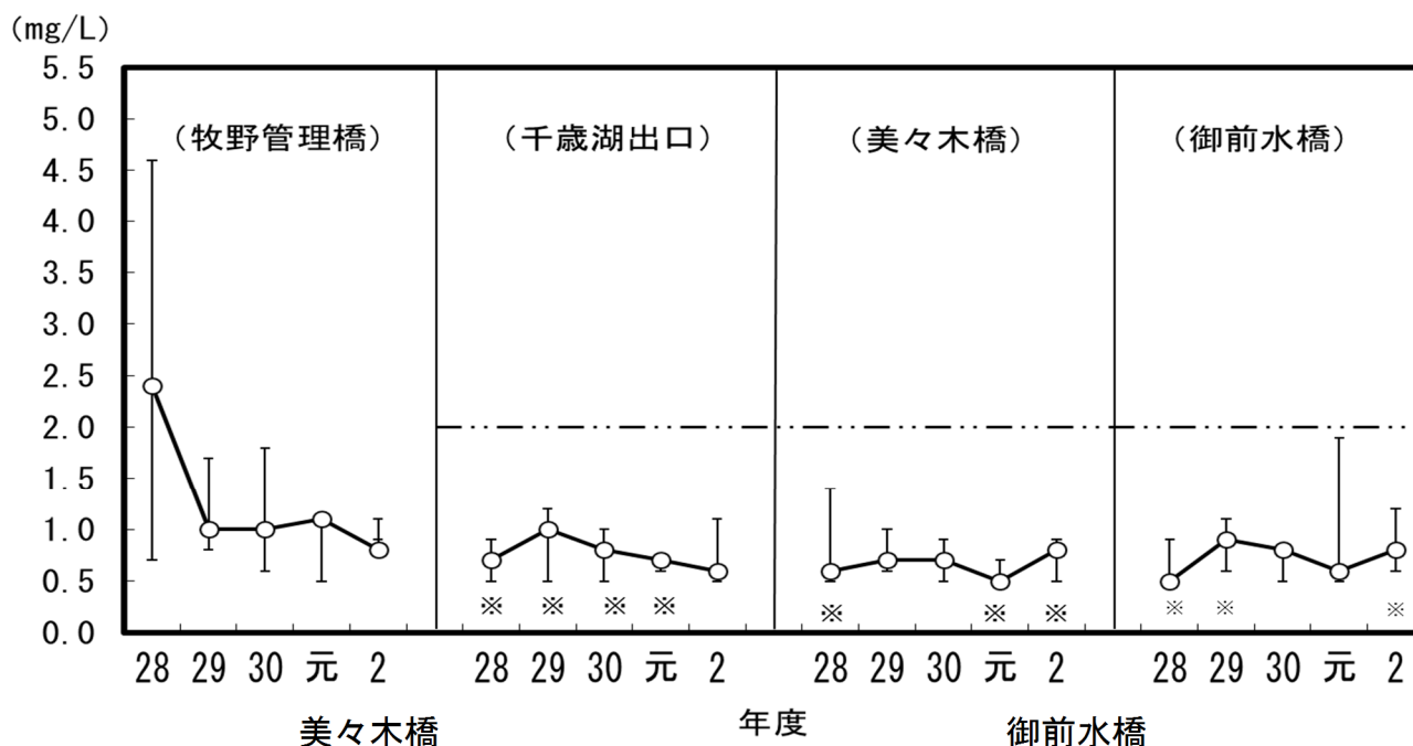
図3-9 BODの経年変化(美々川水系)
