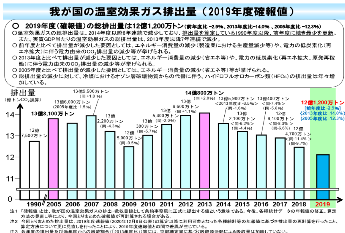
図 1 我が国の温室効果ガス排出量（2019 年度確報値）
