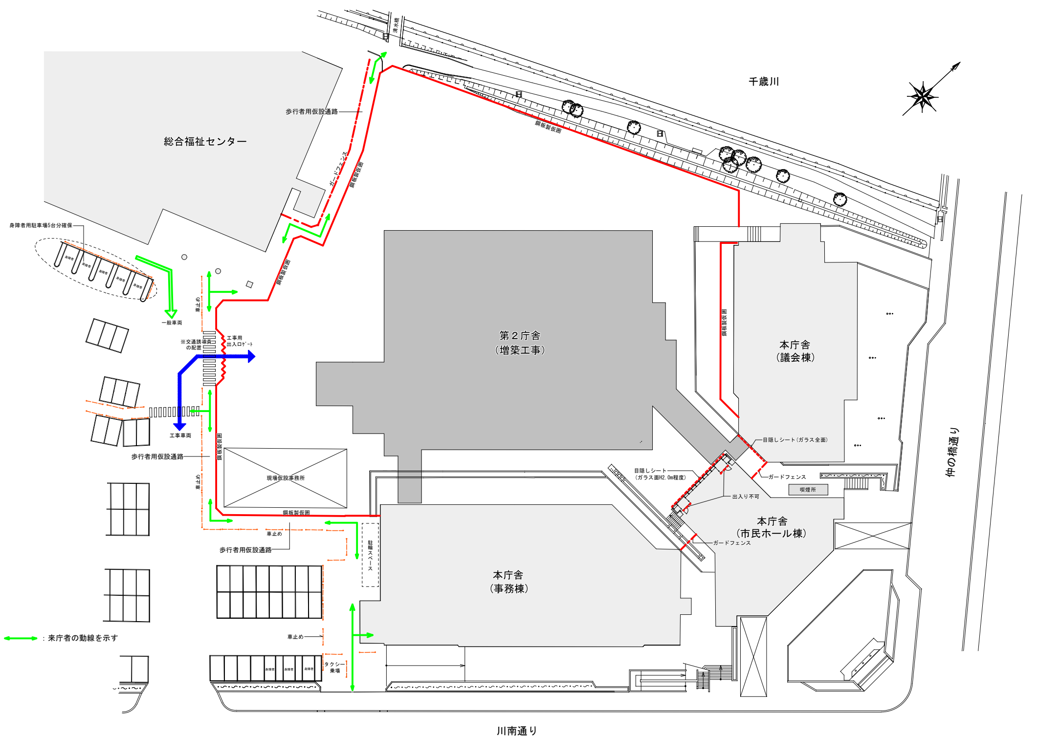
【千歳市第2庁舎建設工事 仮設計画図】
