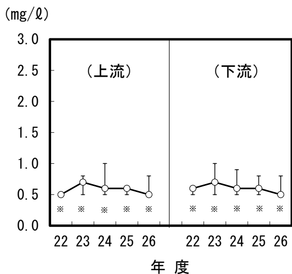
図3-8 BODの経年変化(ママチ川)
