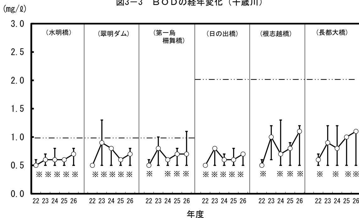
図3-3 BODの経年変化(千歳川)
