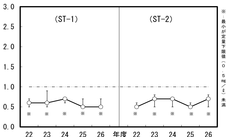
図3-11 CODの経年変化(支笏湖) 26年度は速報値 (mg/ℓ)
