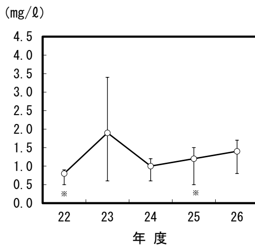
図3-7 BODの経年変化(嶮渚川)
