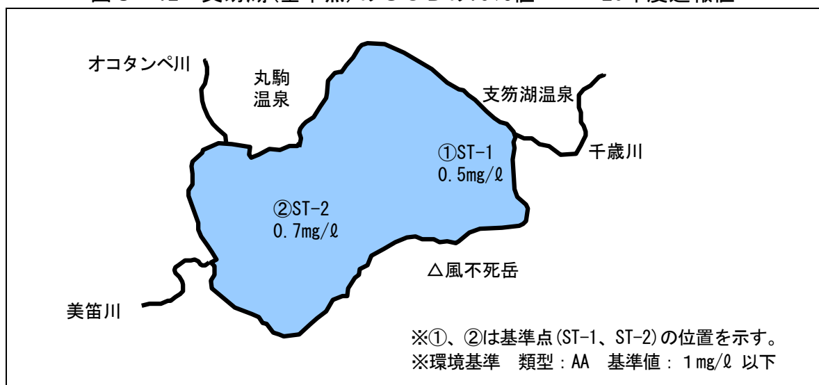
図3-12 支笏湖(基準点)のCODの75%値 26年度速報値
