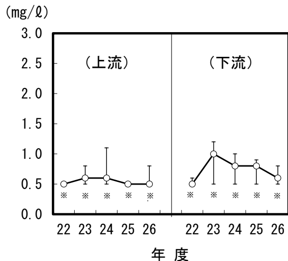
図3-6 BODの経年変化(長都川)
