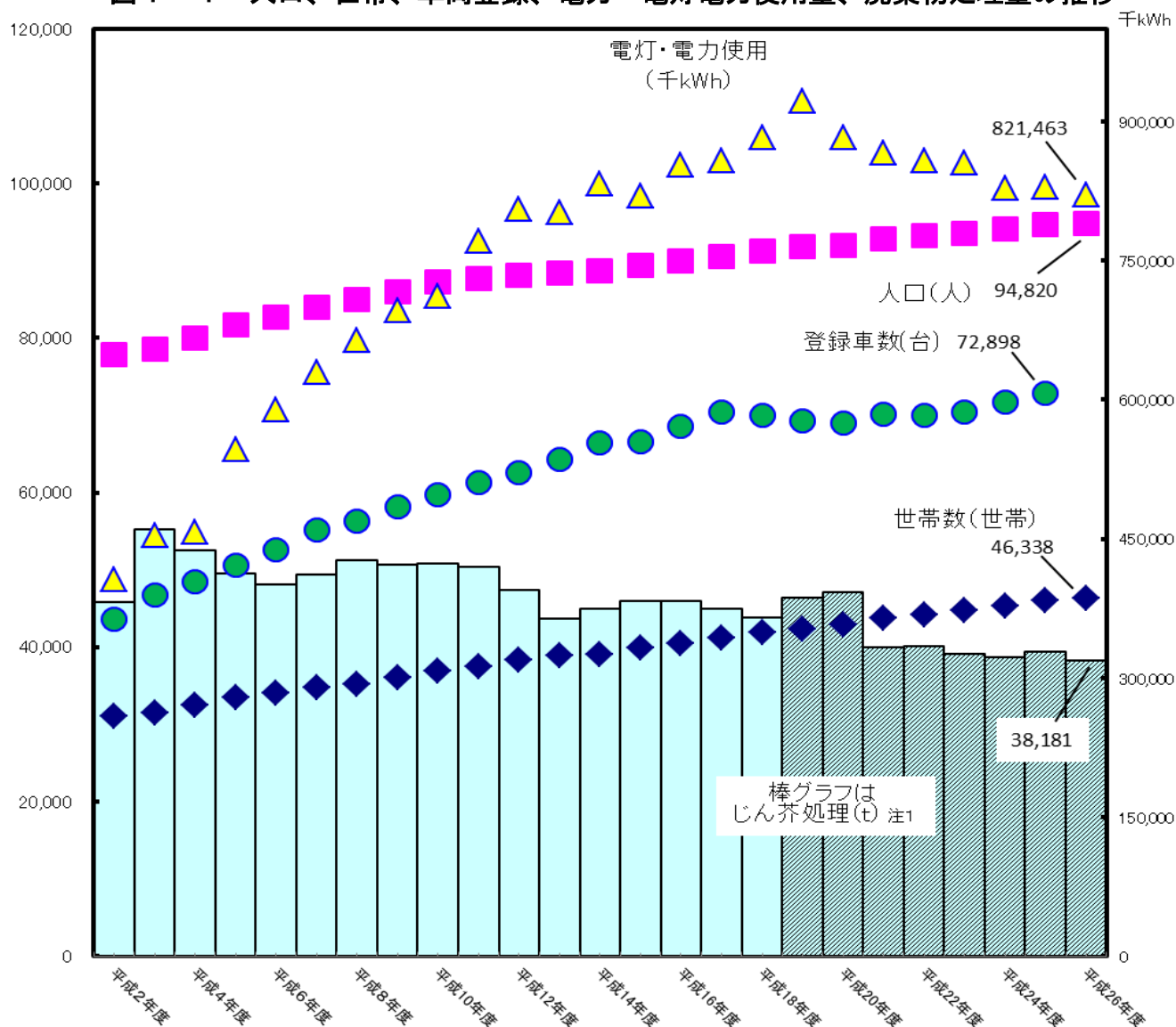
図1-1 人口、世帯、車両登録、電力・電灯電力使用量、廃棄物処理量の推移
