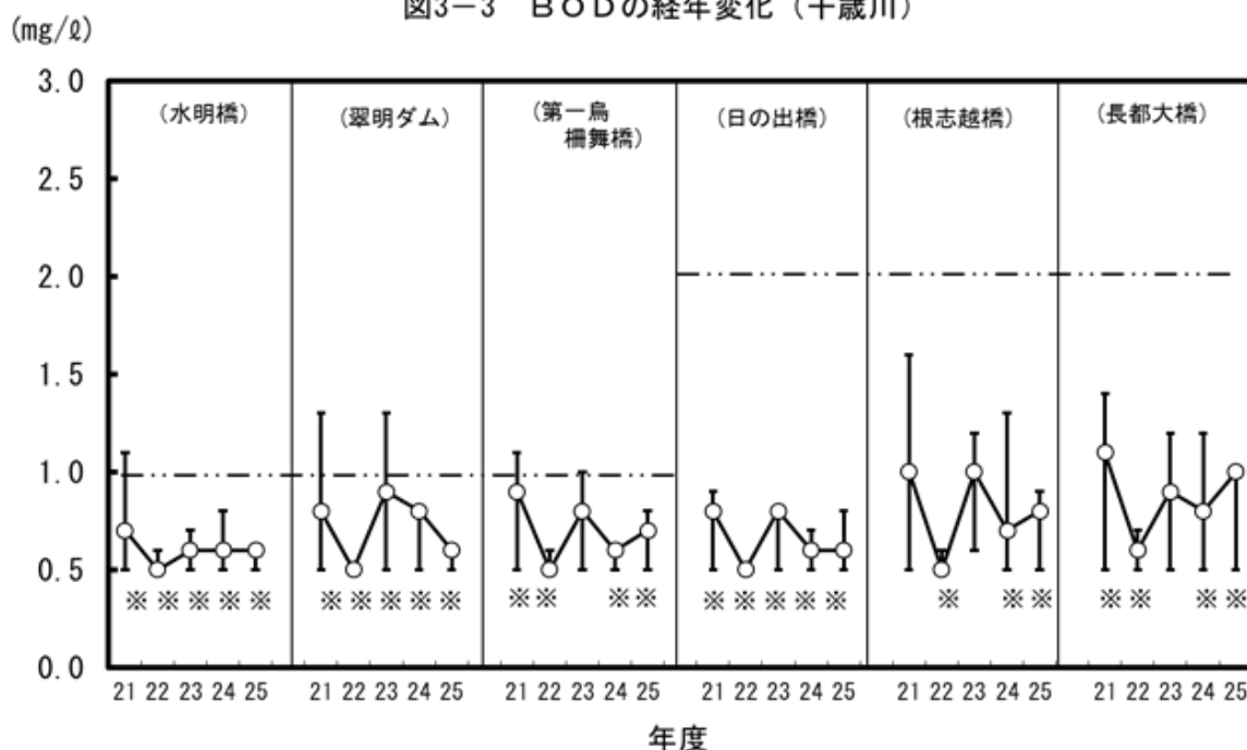
図3-3 BODの経年変化(千歳川)
