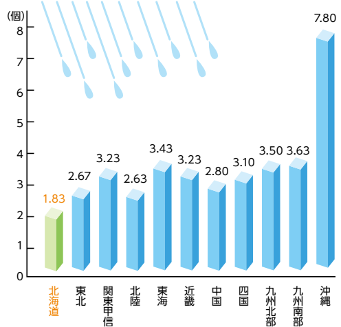
■台風 過去30年間(1985~2014年)の台風年平均接近数
