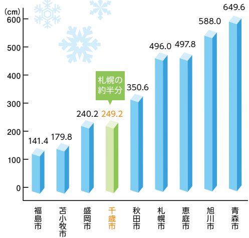
■降雪 国内各都市の年間降雪量(2010~2014年の平均)
