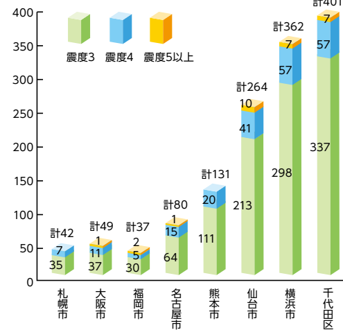
■地震 過去89年間の震度3以上の地震発生回数 (1926年1月1日~2014年12月31日)
