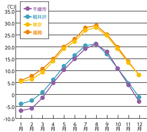
■気温 最近5カ年(2010~2014年)の平均気温比較
