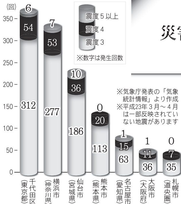
図1：震度3以上の地震発生回数 (大正15年1月～ 平成23年4月の85年間)
