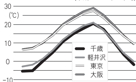
図4：主な都市の月気温(平成18~22年の平均)
