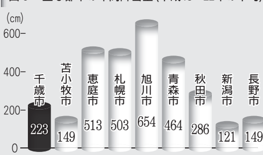
図6：主な都市の年間降雪量(平成18~22年の平均)
