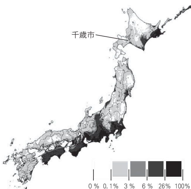
図2：今後30年間に震度6弱以上の地震が発生する確率
