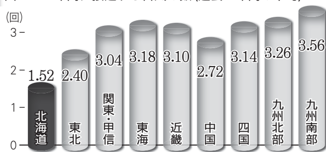
図3：1年間に接近する台風の数(過去50年間の平均)
