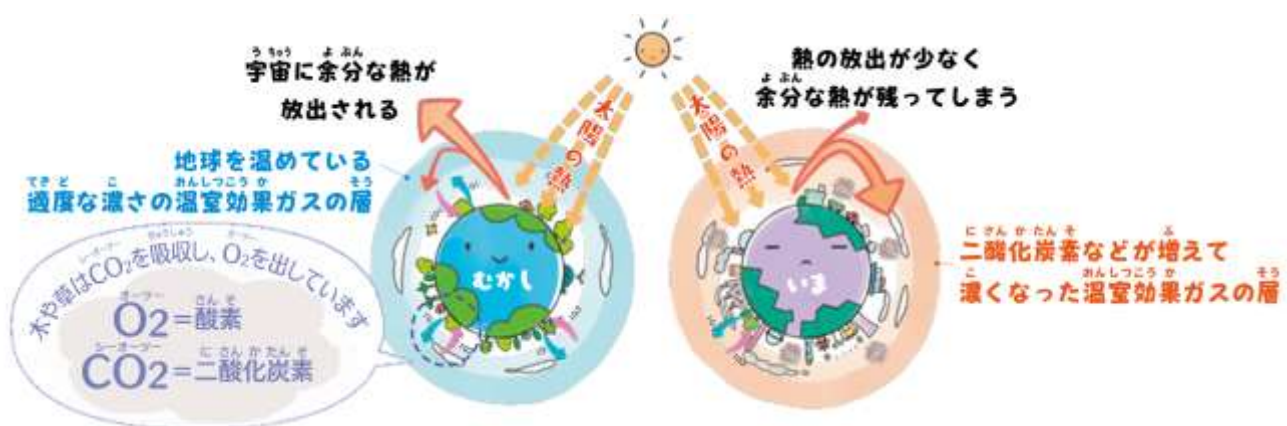
図1-2 地球温暖化の仕組み
