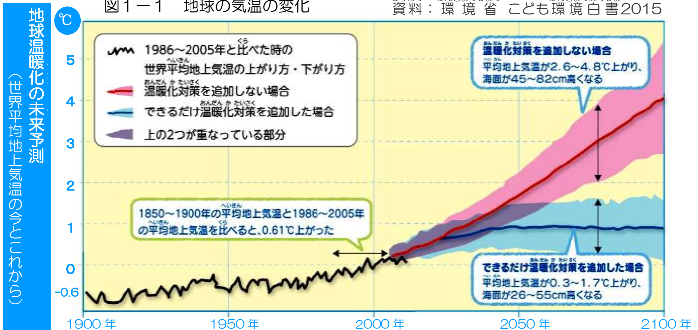
図1-1 地球の気温の変化
