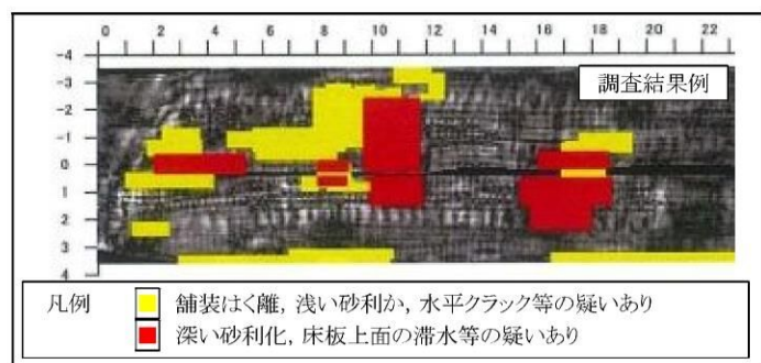
図2 床版解析画像
