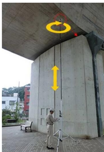
写真9 点検ロボットカメラ による高所点検状況
