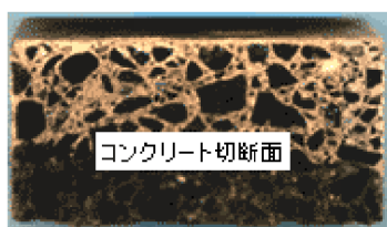
写真15 無溶剤タイプジェル状シラン系表面含浸材
