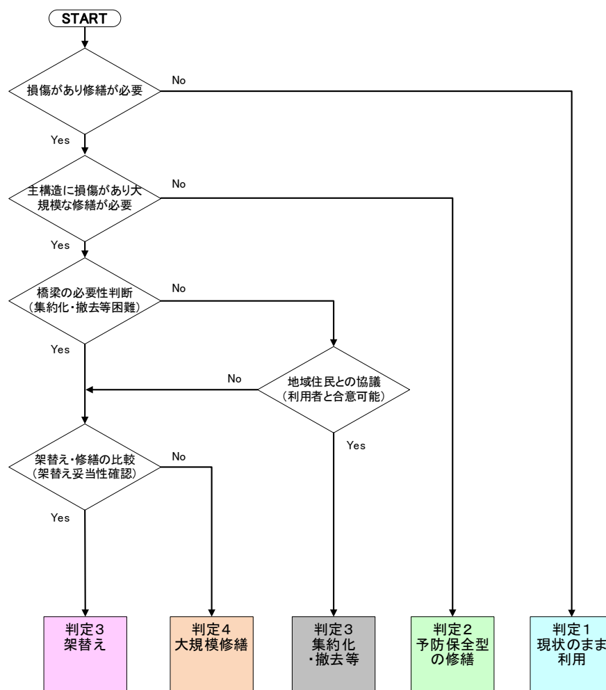
架替え、修繕、集約化・撤去等橋梁選定フロー
