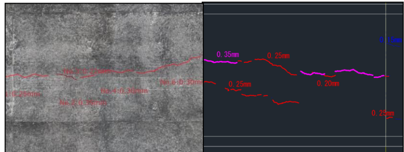
図1 画像解析によるひび割れ図作成
