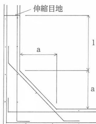
( b ) 平面図
