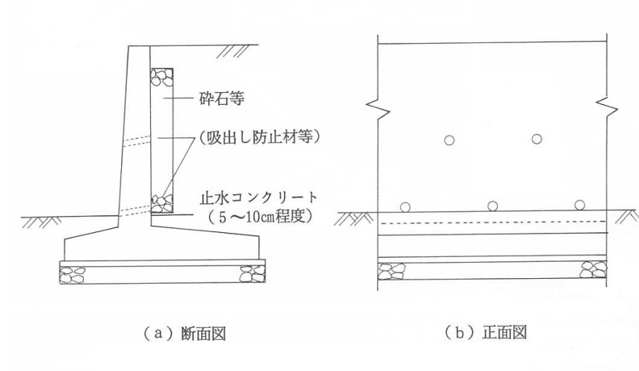
水抜穴の配置図
