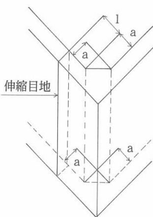
( a ) 立体図
