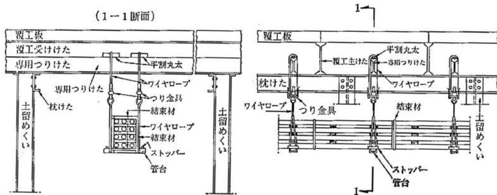
図 5-7 つり防護図
