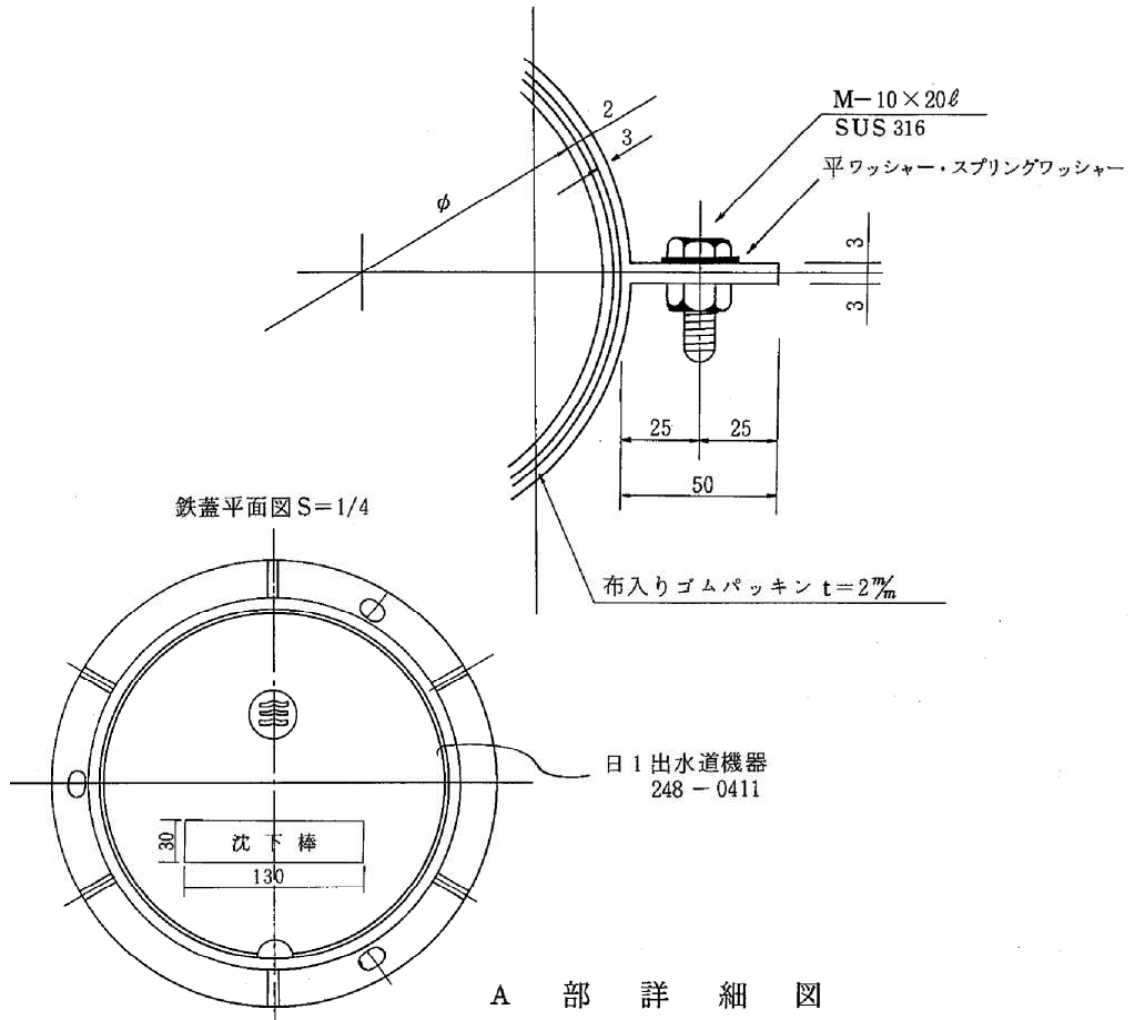
A 部 詳 細 図 S=1/2
