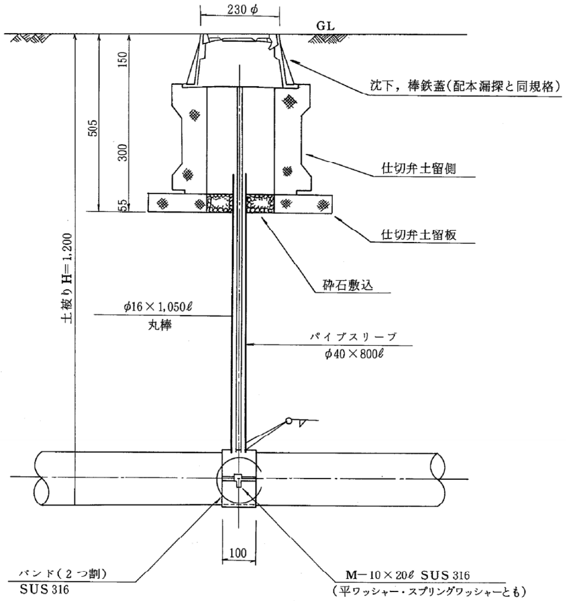
断面図 S = 1/10
