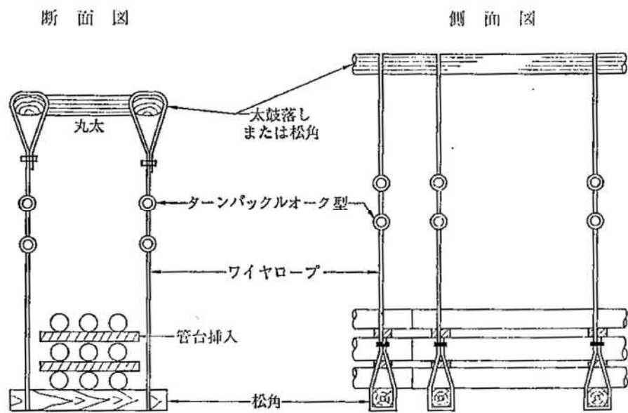
図 5-9 つり防護図
