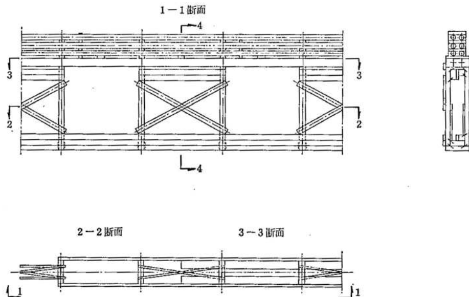
図 5-8 受け防護図
