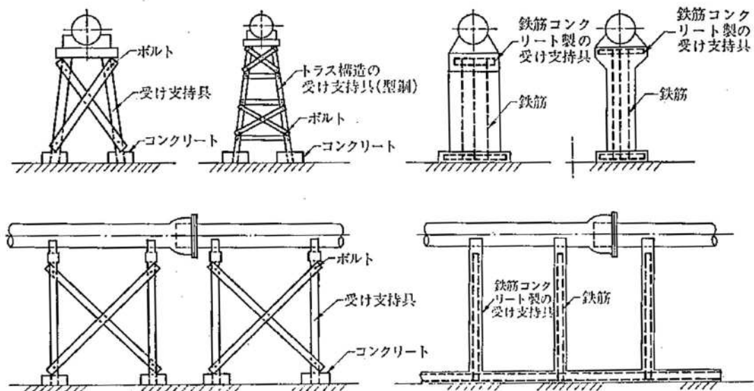
図 5-2 受け防護図
