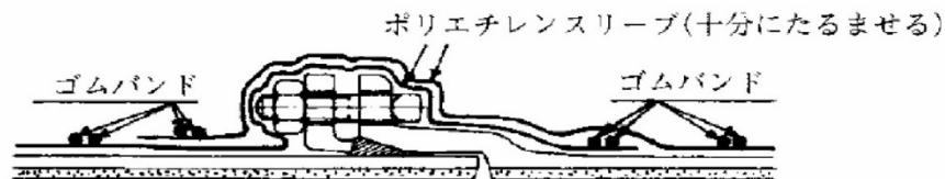
図-48 A法による継手部施工詳細図
