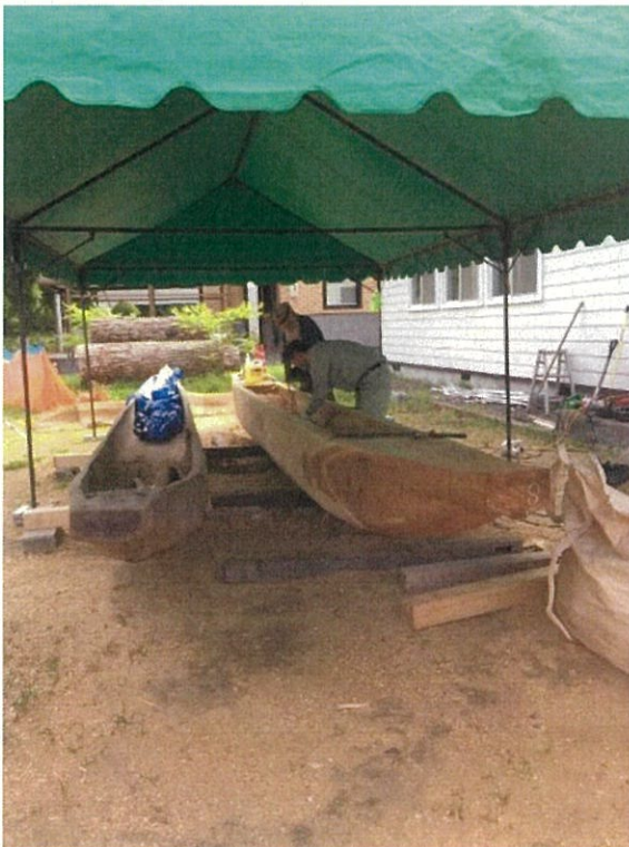
令和3年7月9日 船体内部削り(中盤)(30年前に制作したチプを並べて参考にしながら作業)
