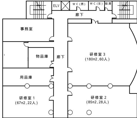
3階 平面図
