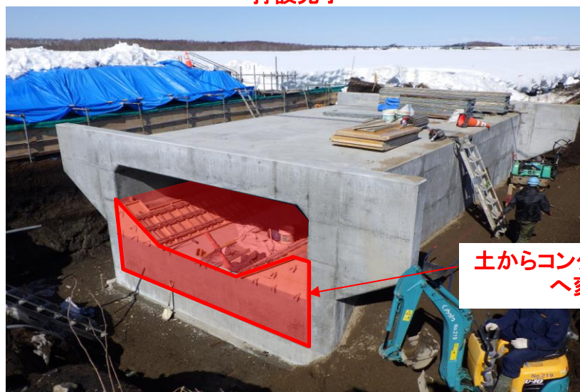
打設完了
